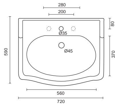
Cod. 3070 Lavabo su colonna / Washbasin on pedestal Cod. 3080 Colonna in ceramica / Ceramic pedestal
