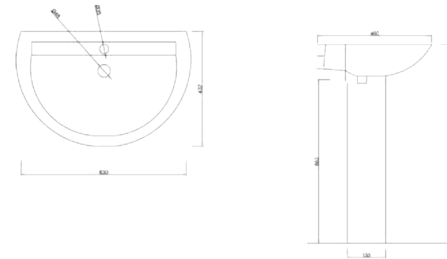
Cod. BELA103 Lavabo sospeso o su colonna / Wall-hung or pedestal washbasin Cod. BELA102 Lavabo sospeso o su colonna / Wall-hung or pedestal washbasin Cod. BECO104 Colonna in ceramica / Ceramic pedestal
