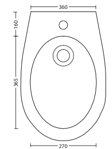
Cod. W0204 Bidet sospeso / Wall hung bidet
