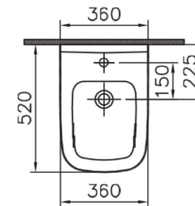
Cod. 5508L003-1046 Bidet sospeso / Wall hung bidet
