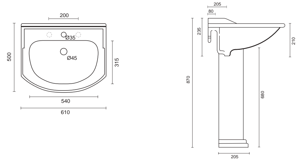
Cod. 3180 Lavabo su colonna / Washbasin on pedestal Cod. 3200 Colonna in ceramica / Ceramic pedestal
