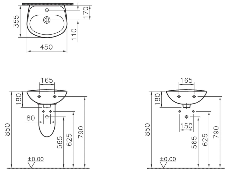
Cod. 5078L003-001 Lavabo 45 sospeso o su semicolonna / Wall-hung or semi-pedestal washbasin 45
