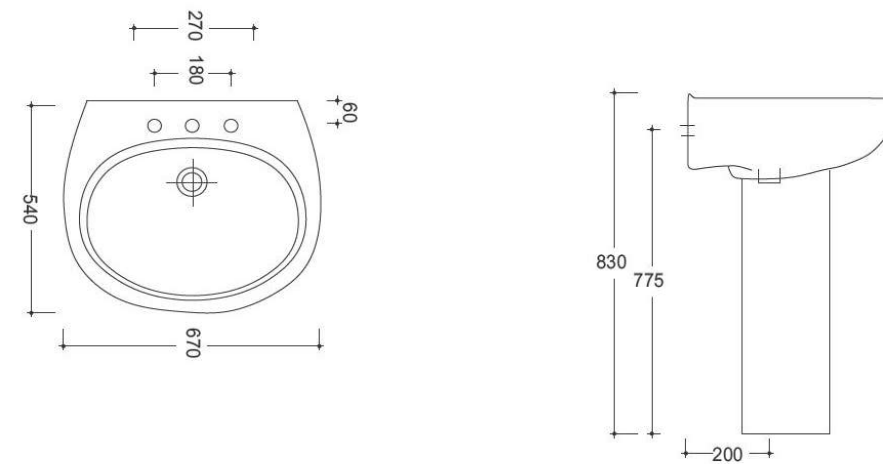
Cod. 00200 Lavabo su colonna / Washbasin on pedestal Cod. 00201 Colonna in ceramica / Ceramic pedestal
