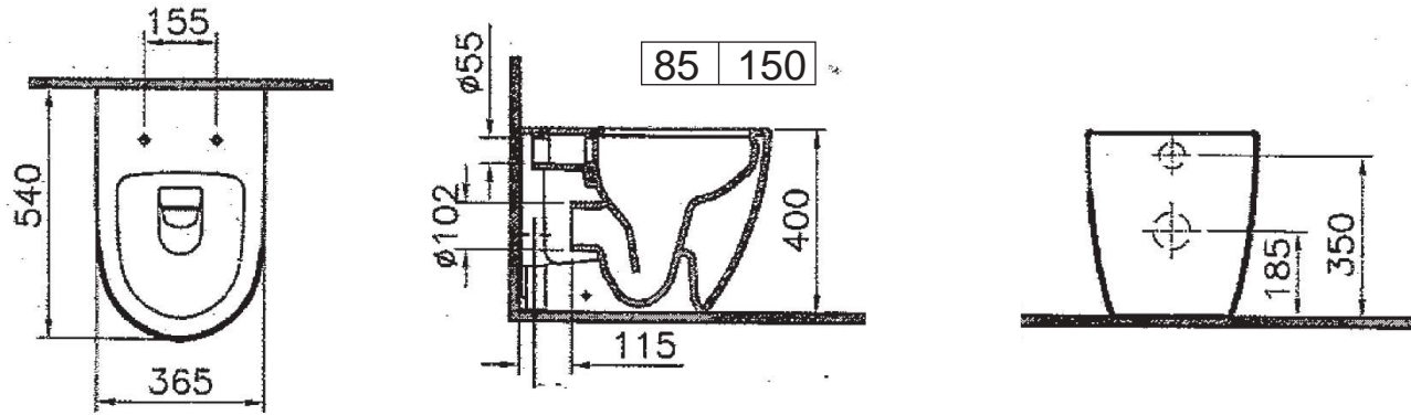
Cod. 7985B003-0075 WC a terra rimless trasformabile tramite curva tecnica / Rimless back to wall WC, adjustable by elbow/wall pipe
