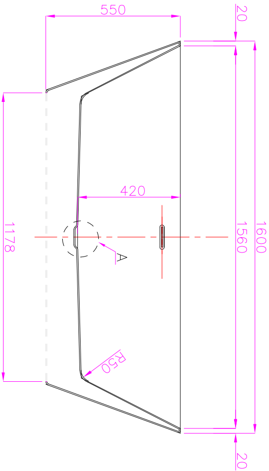
SEZIONE F-F
