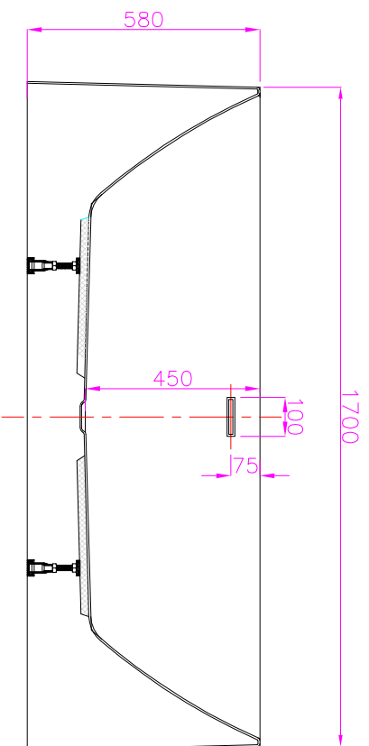
SEZIONE G-G
