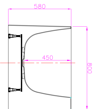
SEZIONE F-F
