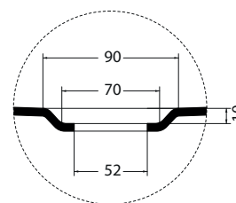
DETTAGLIO C
