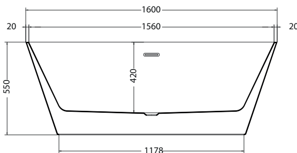
SEZIONE A-A'
