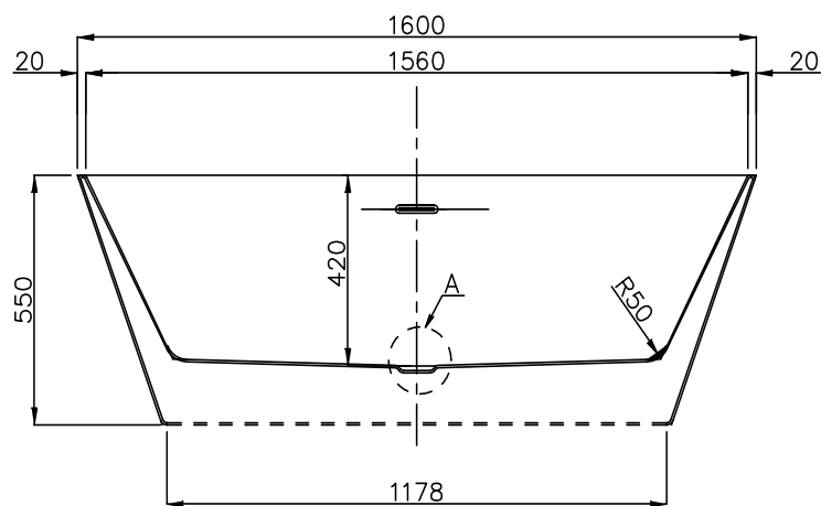
SEZIONE F-F
