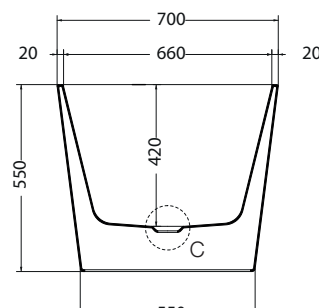
SEZIONE B-B'
