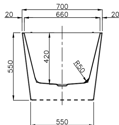
SEZIONE G-G
