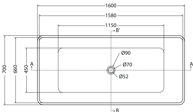
PIANTA
