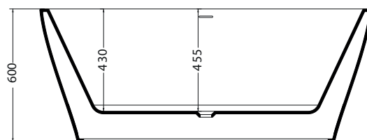
SEZIONE A-A'
