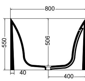
SEZIONE B-B'
