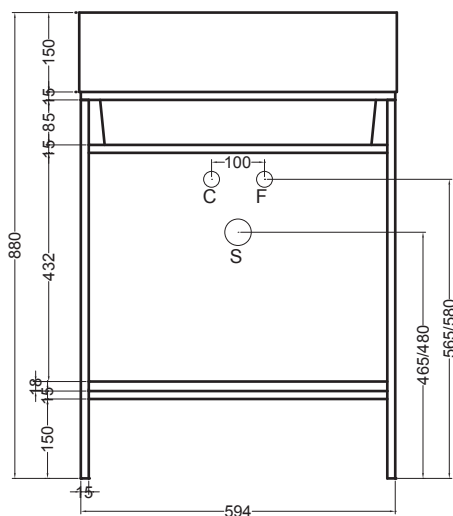
VISTA FRONTALE
