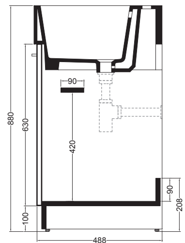
VISTA IN SEZIONE B-B
