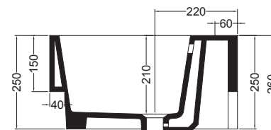
SEZIONE B-B
