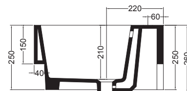
SEZIONE B-B
