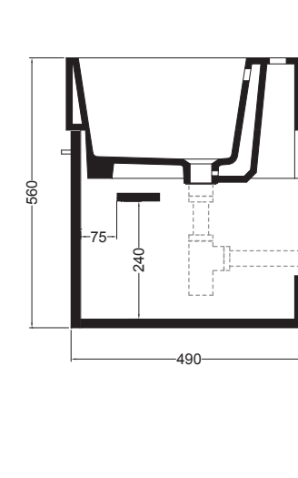
VISTA IN SEZIONE B-B
