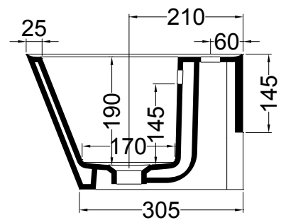
SEZIONE A-A'
