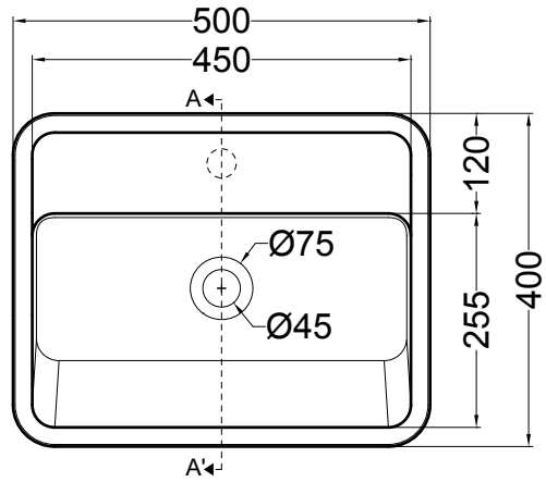
PIANTA
