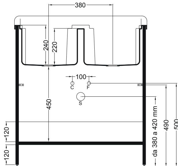
SEZIONE A-A'
