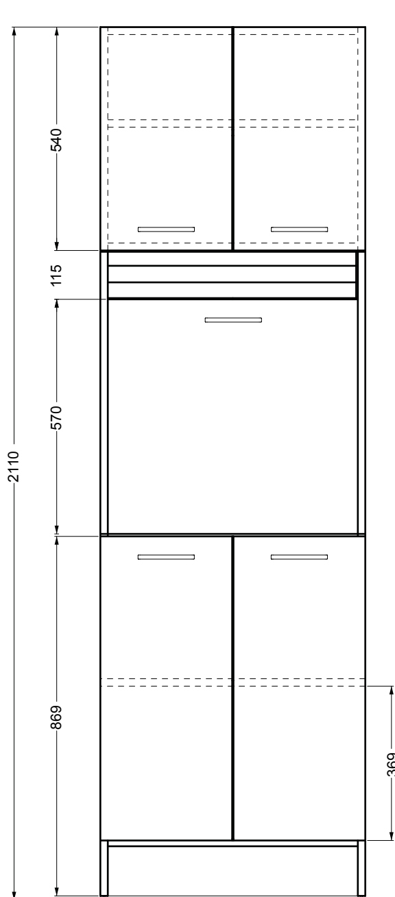
VISTA FRONTALE
