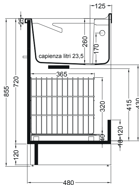
SEZIONE A-A'
