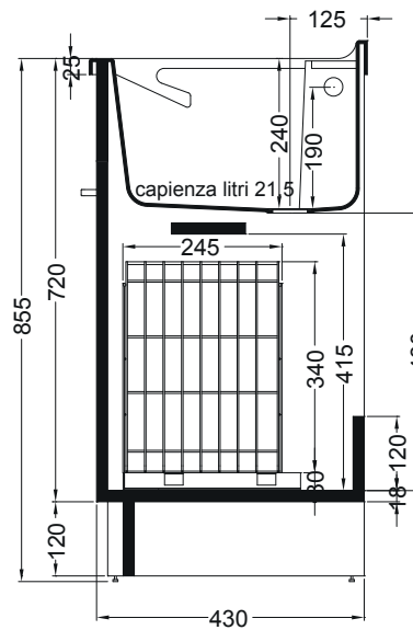
SEZIONE A-A'
