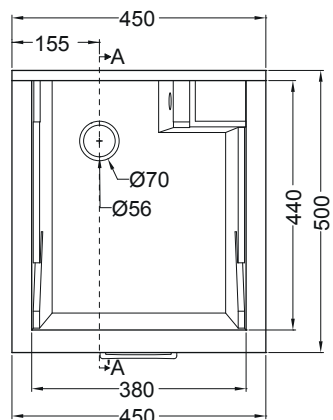
PIANTA
