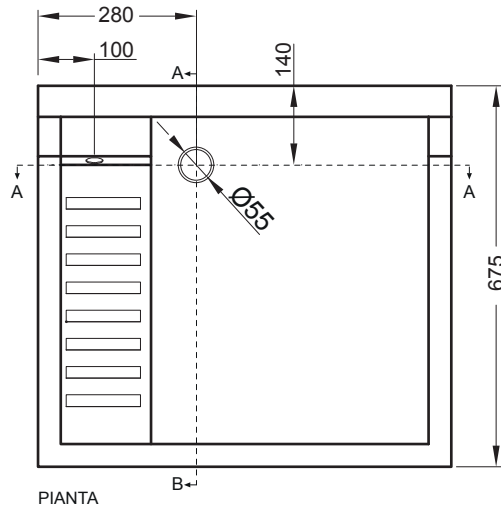
PIANTA
