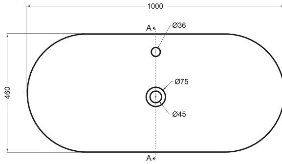
PIANTA PLAN
