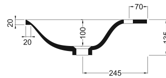
SEZIONE A-A SECTION A-A
