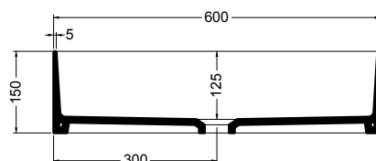
SEZIONE
