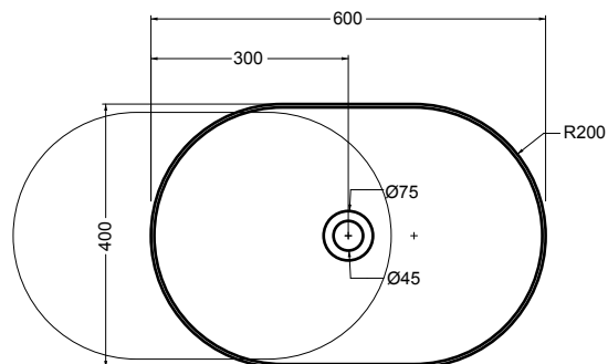
PIANTA
