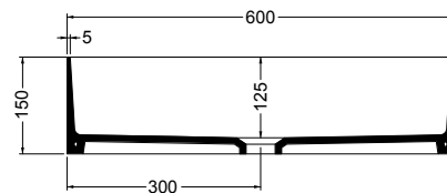
SEZIONE
