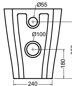
VISTA POSTERIORE
