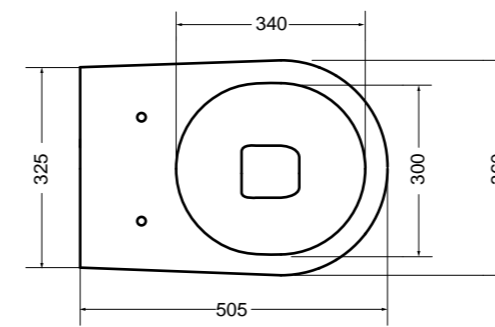
84022 bidet a terra_BTW bidet
