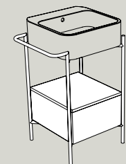
STRUTTURA/CASSETTO FRAME/DRAWER S864807/MSC420 58x48xh80 cm
