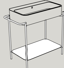
STRUTTURA/RIPIANO FRAME/SHELF S8610007/R8610007 110x45xh80 cm
