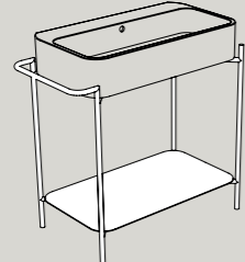
STRUTTURA/RIPIANO FRAME/SHELF S868007/R868007 90x45xh80 cm
