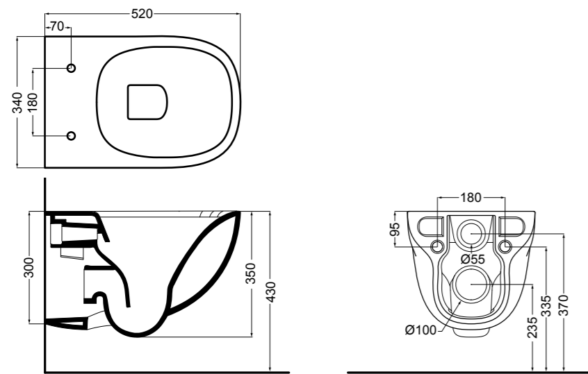
30060 vaso sospeso NORIM®_wall hung wc NORIM®
