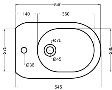
PIANTA PLAN
