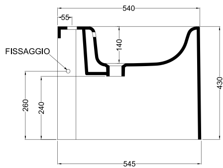
SEZIONE LONGITUDINALE LONGITUDINAL VIEW
