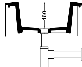
SEZIONE TRASVERSALE CROSS VIEW
