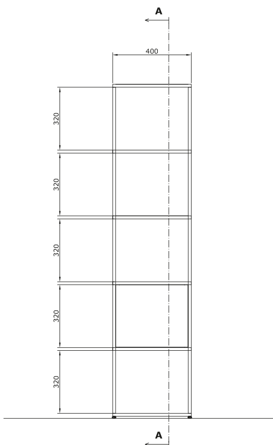
VISTA FRONTALE
