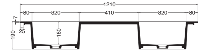
SEZIONE LONGITUDINALE
