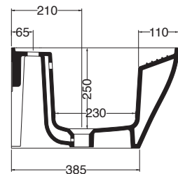
SEZIONE TRASVERSALE
