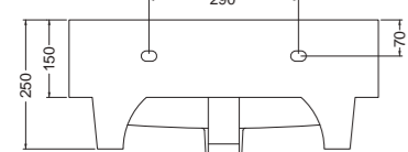
VISTA POSTERIORE
