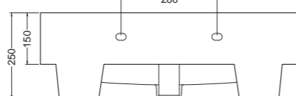
VISTA POSTERIORE
