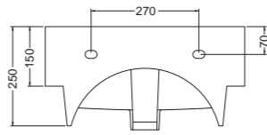
VISTA POSTERIORE
