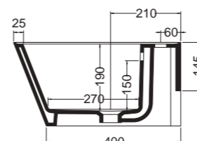
SEZIONE TRASVERSALE
