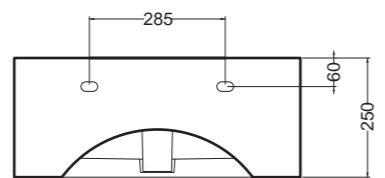
VISTA POSTERIORE
