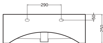
VISTA POSTERIORE
