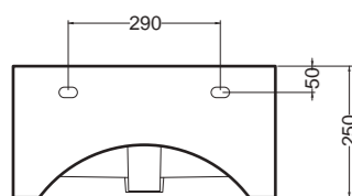
VISTA POSTERIORE
