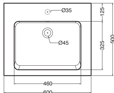
PIANTA
