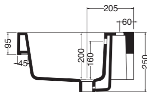
SEZONE TRASVERSALE
