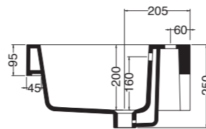
SEZONE TRASVERSALE
