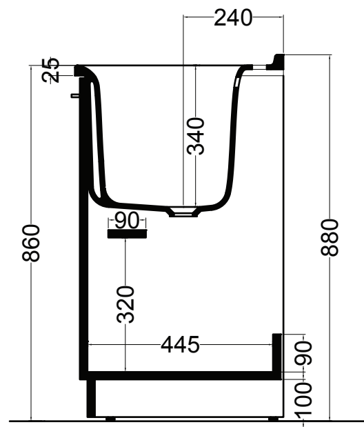
SEZIONE A-A
