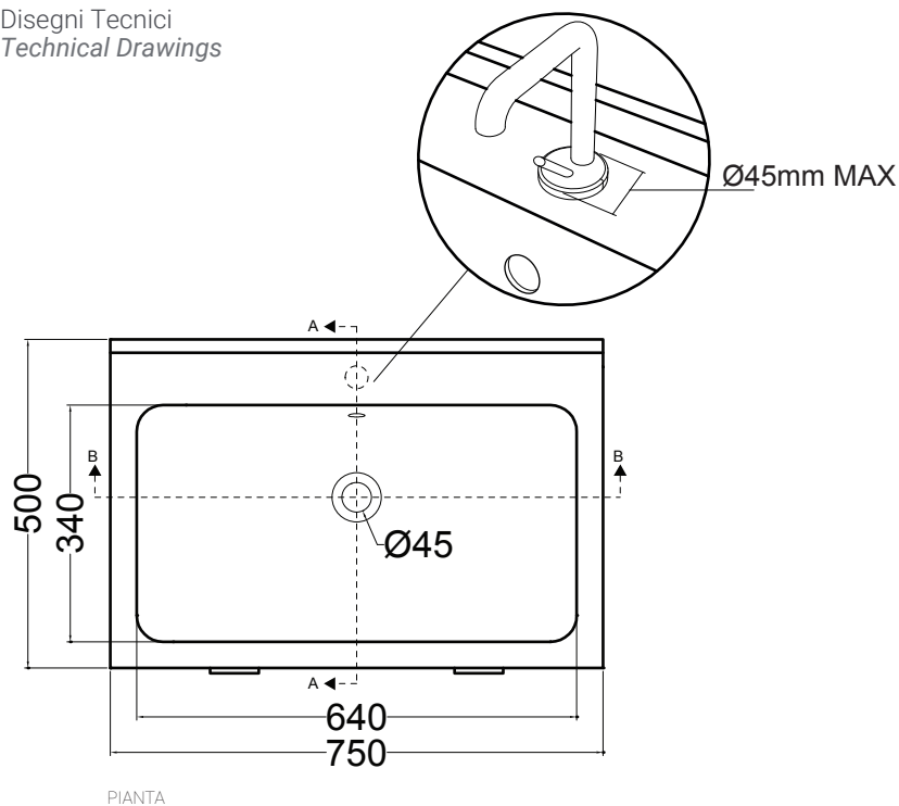
PIANTA
