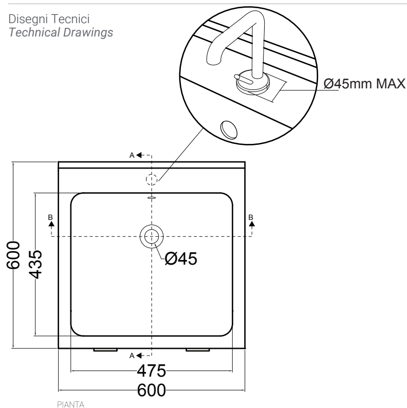
PIANTA
