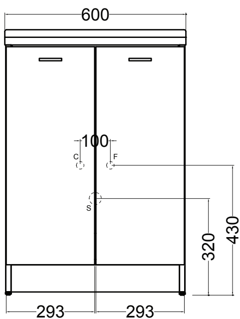
VISTA FRONTALE
