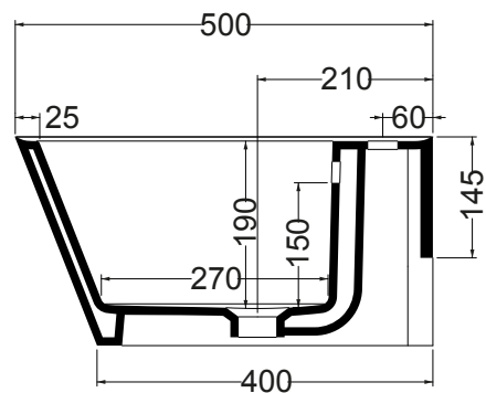
SEZIONE A-A'
