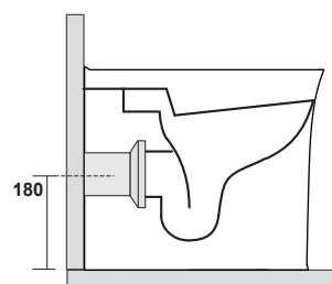
tubo di raccordo a parete art. 7539
