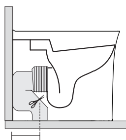
max. 230 // min. 170 con curva art. 7619
