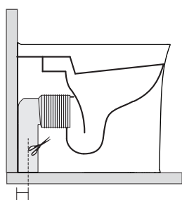
max. 140 // min. 60 con curva art. 900104
