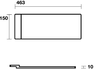
7814 Pianetto per lavabo Kanaal cm 60 (5740) Shelf for Kanaal washbasin cm 60 (5740)
