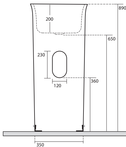
VERSIONE SCARICO PARETE
