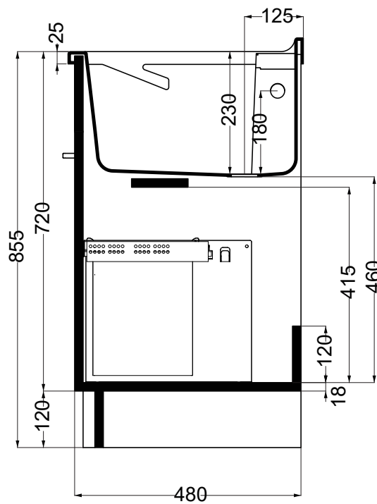
SEZIONE A-A'
