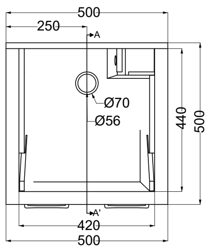
PIANTA
