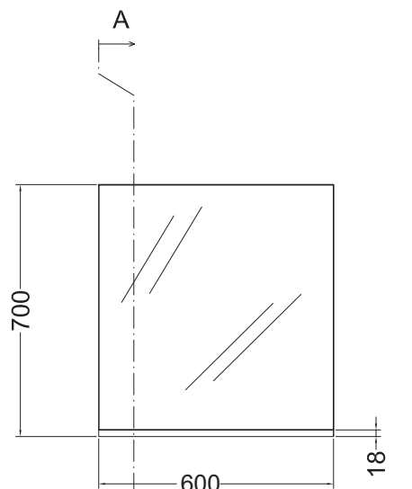
VISTA FRONTALE
