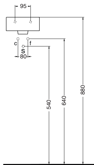
VISTA POSTERIORE
