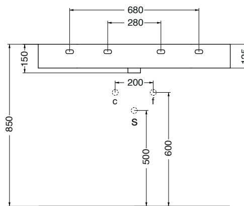
VISTA POSTERIORE
