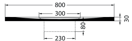
SEZIONE B-B'
