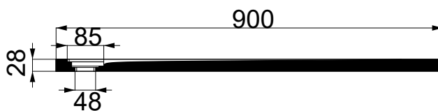
SEZIONE A-A
