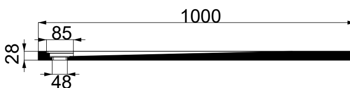
SEZIONE A-A
