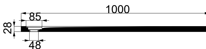
SEZIONE A-A
