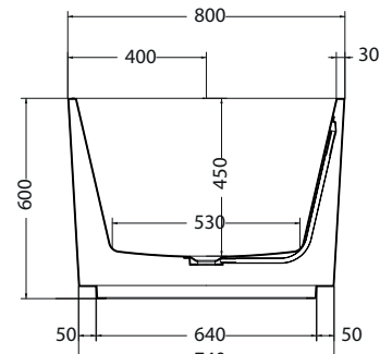
SEZIONE B-B'
